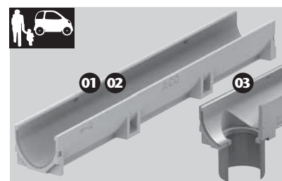
ACO Euroline gootelement (rechts met onderuitlaat)
